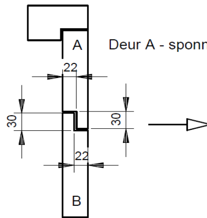
Boerderijdeur type 1
