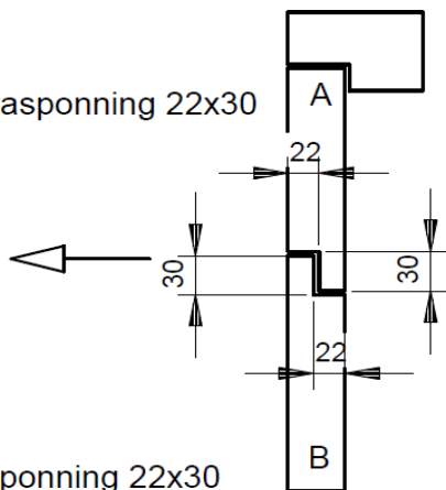
Boerderijdeur type 2
