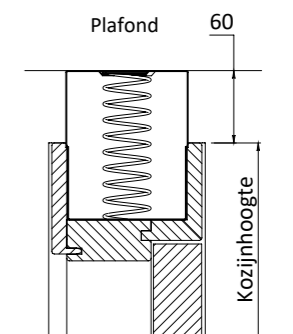
Maximale uitslag Flexunit
