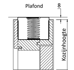
Minimale uitslag Flexunit
