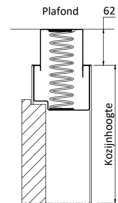
Maximale uitslag Flexunit
